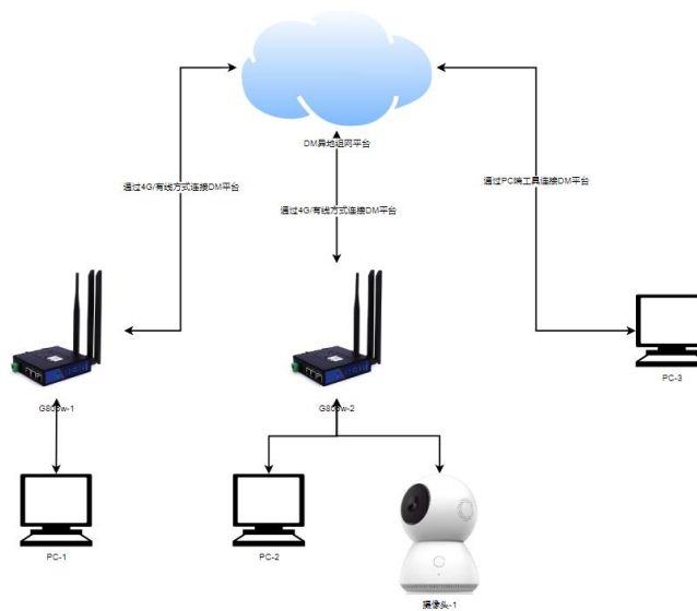
图 5 组网拓扑
