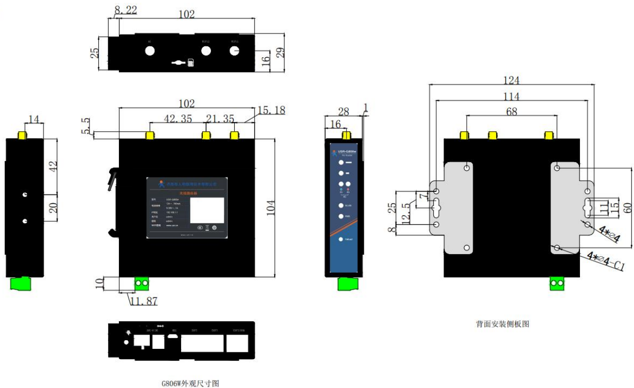
图 1 USR-G806w 尺寸图
