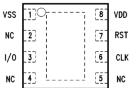
图 24 C2x2eSIM 芯片管脚示意 (TOP VIEW)
