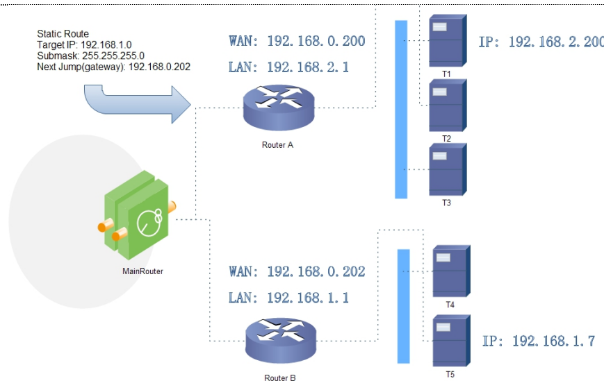
图 42 静态路由表实例图
