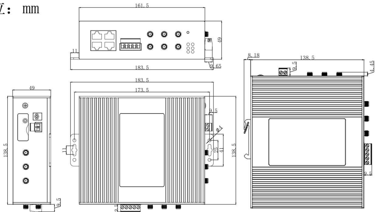
图 1 USR-G817 尺寸图
